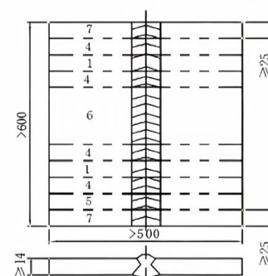
(b) 取侧弯试样时
