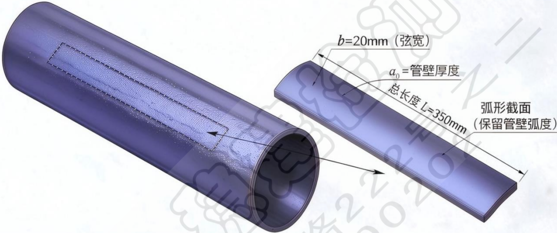
排水铸铁管纵向弧形试样加工图（S3）
